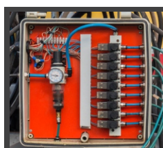
Fijaciones y conexiones eléctricas y neumáticas idem a tablero original para rápida y sencilla instalación.
