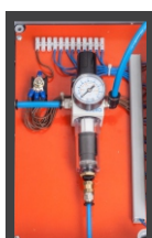
Regufiltro con vaso auto-limpiante.
